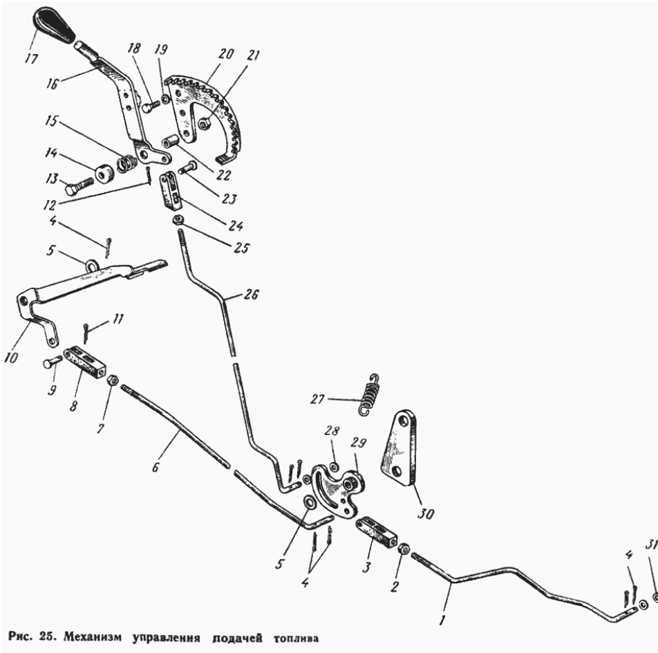
Рис. 25. Механизм управления подачей топлива.
